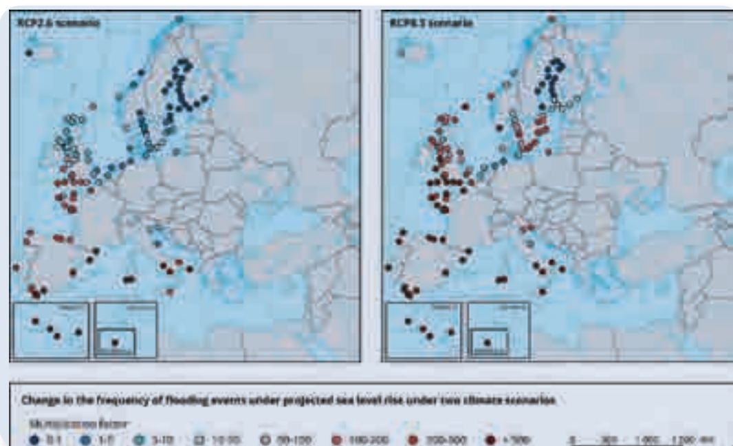
Figure 108 : Evolution de la fréquence des inondations en Europe entre 2010 et 2100 sous la hausse prévue du niveau de la mer, selon deux scénarii de basses (à gauche) et hautes (à droite) émissions (Source : Agence européenne de l'environnement, 2020, adapté du GIEC, 2019)
